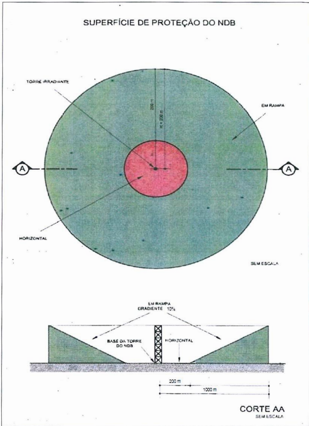
Figura C-2: Superfície de proteção do NDB
