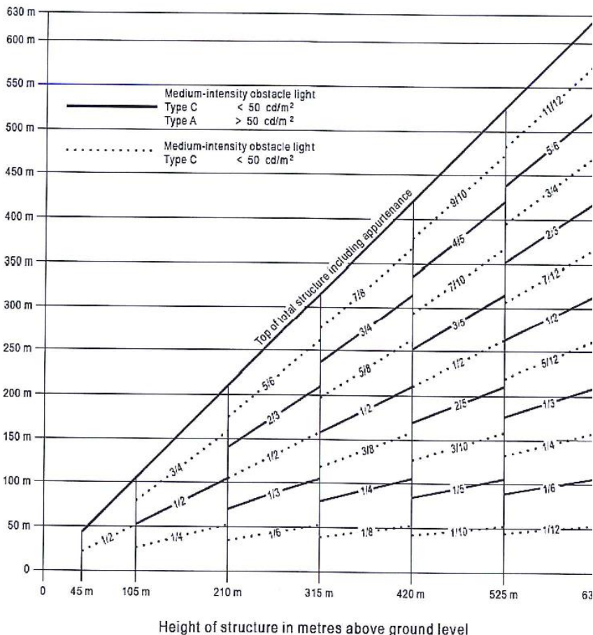
Figura A-5: Sistema duplo de iluminação de obstáculos de média intensidade Tipo A / Tipo C
