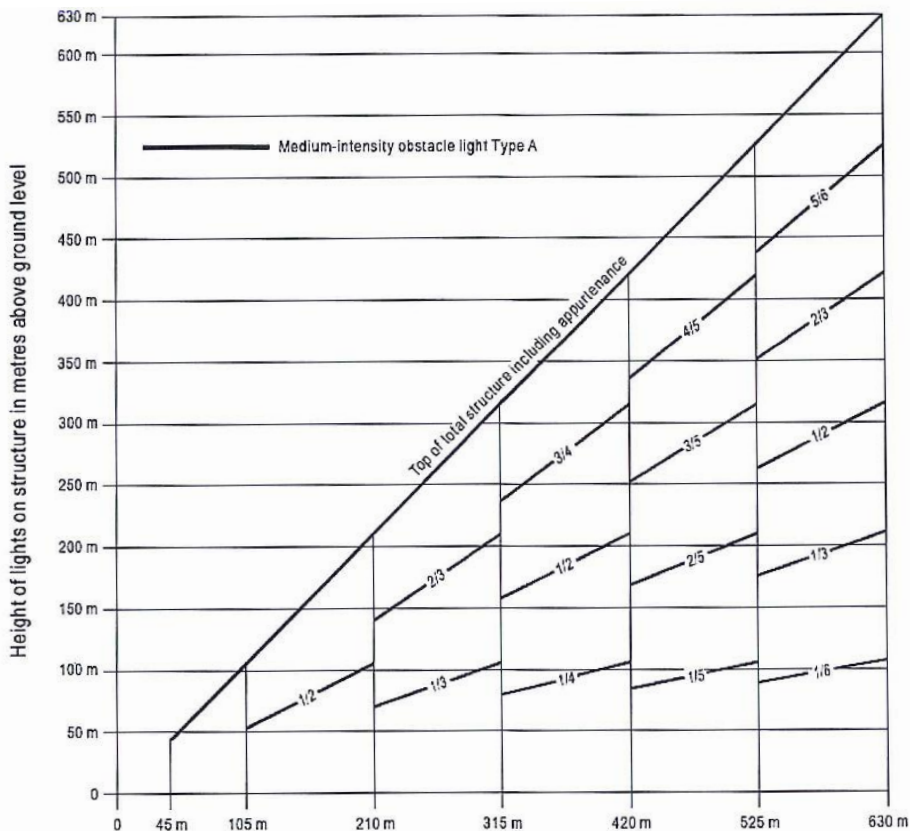
Figura A-1: Sistema de iluminação de obstáculos de média intensidade com luzes brancas intermitentes, Tipo A
