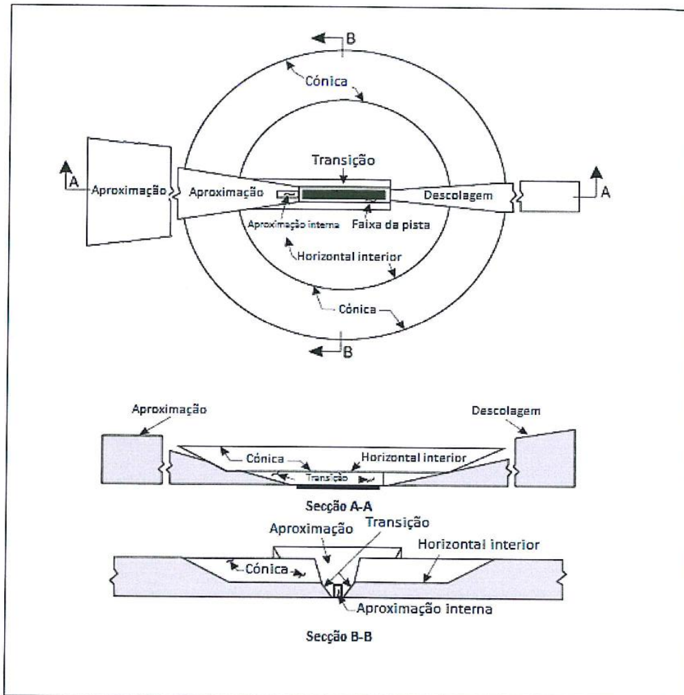
Figura B-1: Superfícies limitadoras de obstáculos
