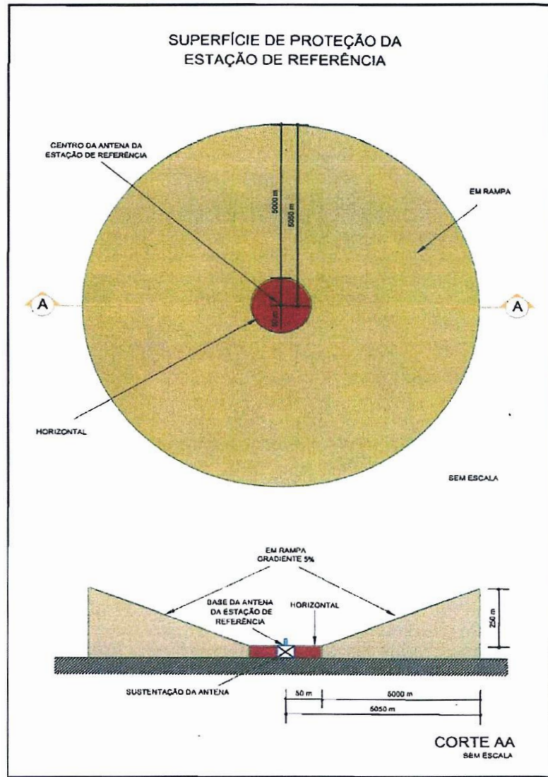
Figura C-5.2: Superfície de proteção da Estação de Referência
