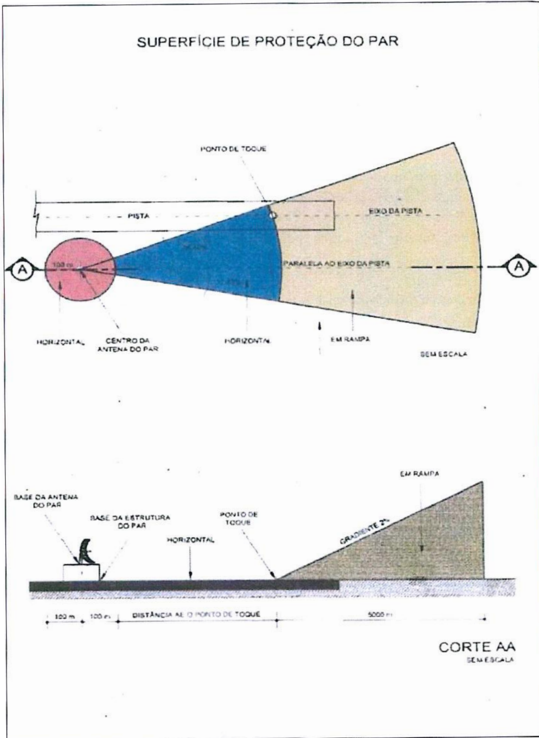
Figura C-9: Superfície de proteção do PAR
