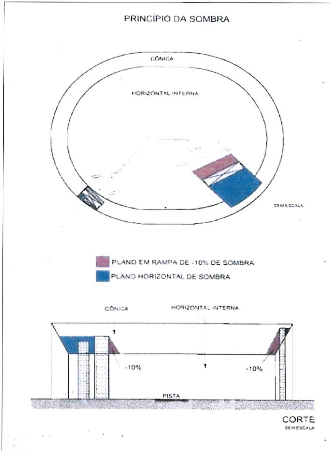
Figura F-1.2: Princípio de sombra
