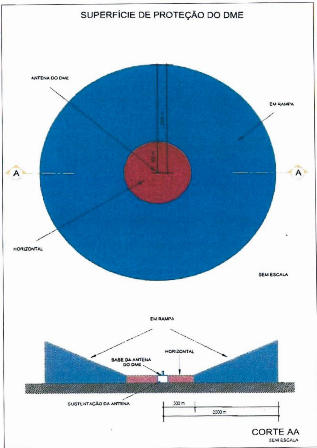
Figura C-1: Superfície de proteção do DME
