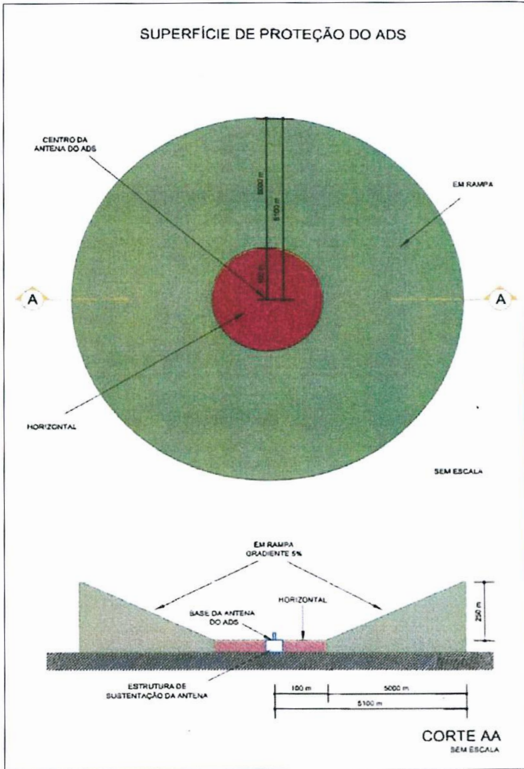
Figura C-10: Superfície de proteção do ADS B
