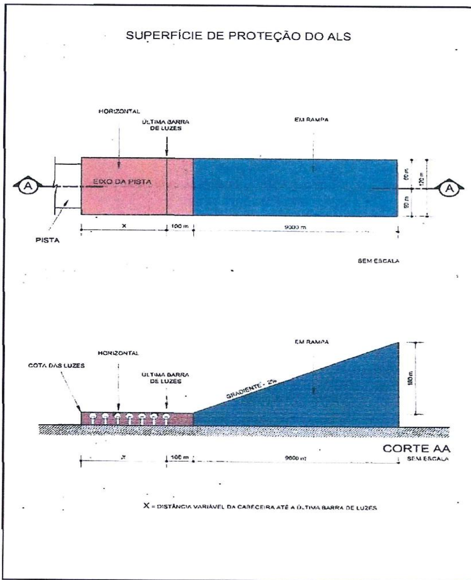
Figura C-6: Superfície de proteção do ALS
