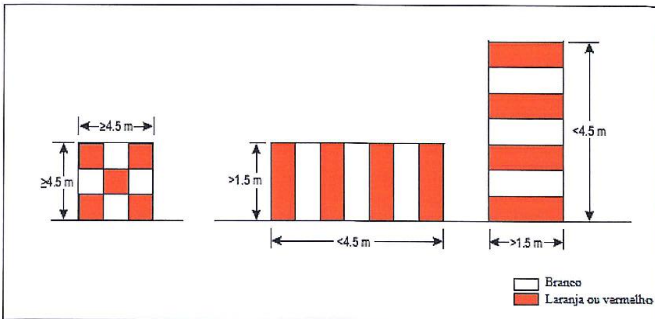
Figura E-1.1: Padrões básicos de sinalização
